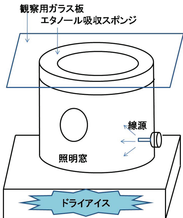
図 8. 自作霧箱の構造
